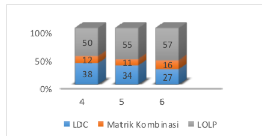
Gambar 3. Waktu Perhitungan N Unit Pembangkit
